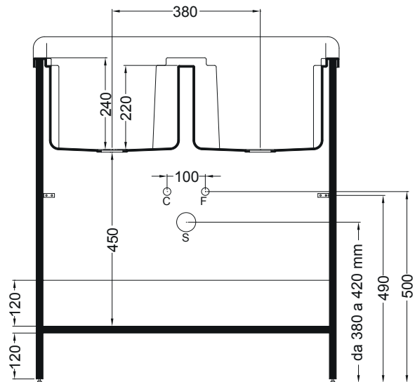
SEZIONE A-A'
